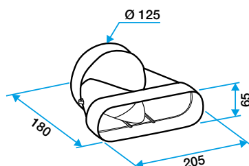
Raccord pour conduit
