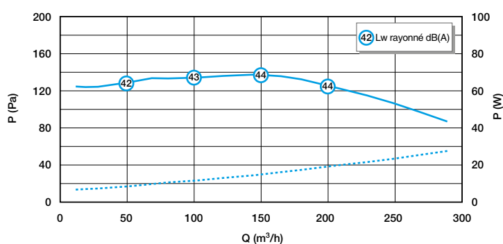
Courbe aérodynamique et acoustique EasyHOME Hygro COMPACT MW
